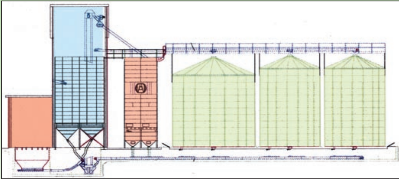
Ritning över anläggningen på Badene. Till vänster finns foderberedningsanläggningen till grisarna.
